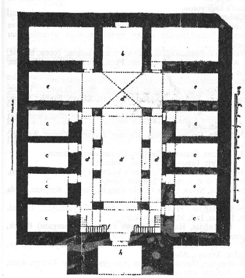
Seraceddin Medresesi Kitâbesi ve Plânı
