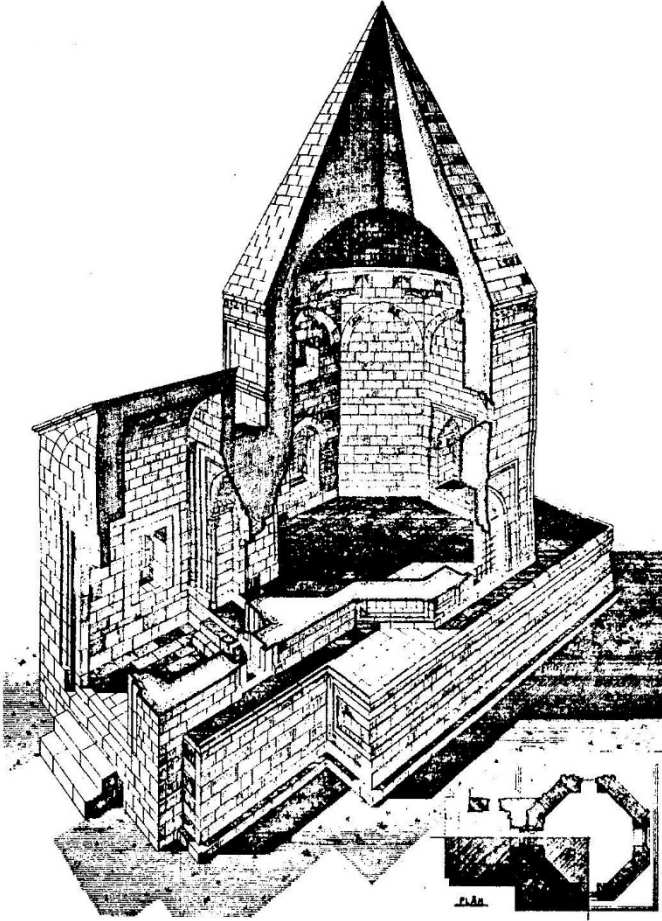
Ali Cafer Kumbeti'nin plân ve kesit görünüşü
