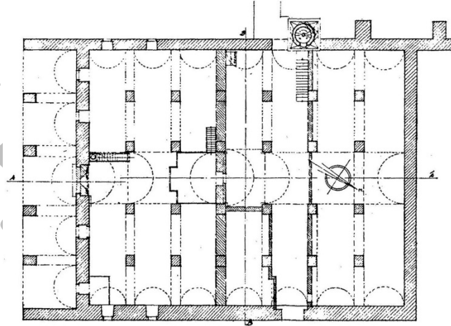
Han Câmî î Plânı
