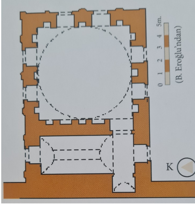
Kütüphane Plâni
